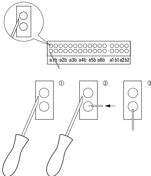
Afbeelding 11: Draad aansluiten op ISDN Homevox.
