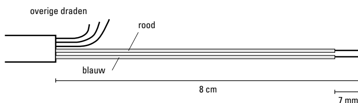
Afbeelding 9: Telefoonkabel strippen.
