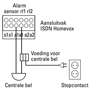
Afbeelding 20: Centrale bel aansluiten.
