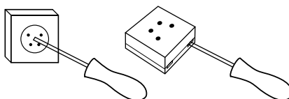
Afbeelding 8: Telefoonstopcontact openen.
