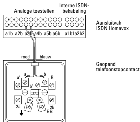
Afbeelding 12: Telefoonkabels van analoge telefoons aansluiten op ISDN Homevox.
